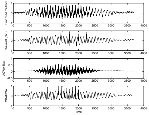
(d) Denoising of noisy signal /i/.
